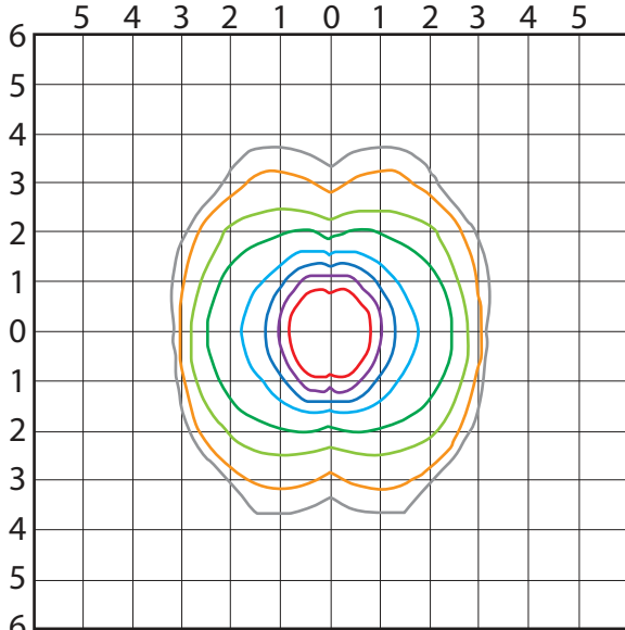
904938 Flex DE Iso Footcandle Plot
