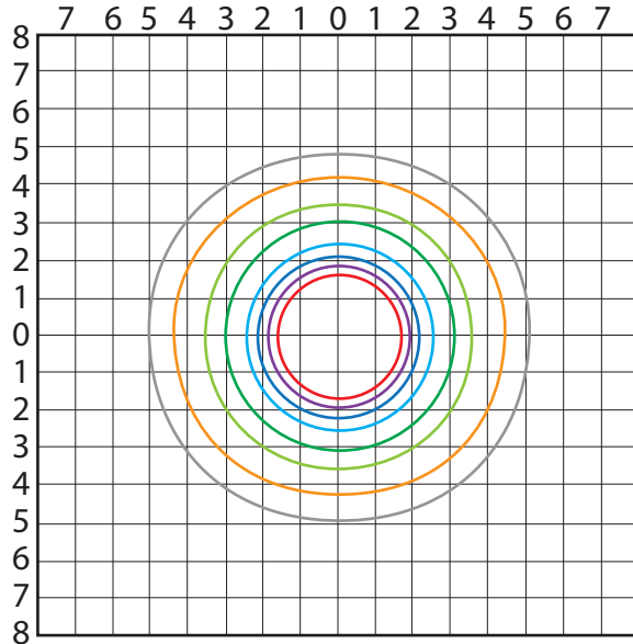
904916 Silver Sun DE Iso Footcandle Plot
